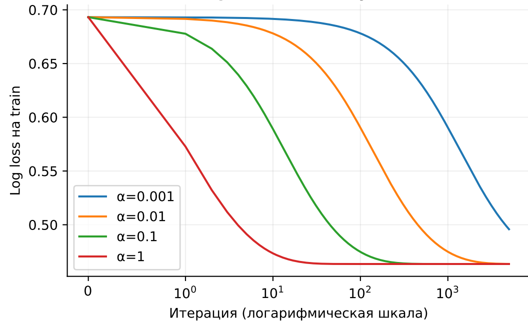
Градиентный спуск
