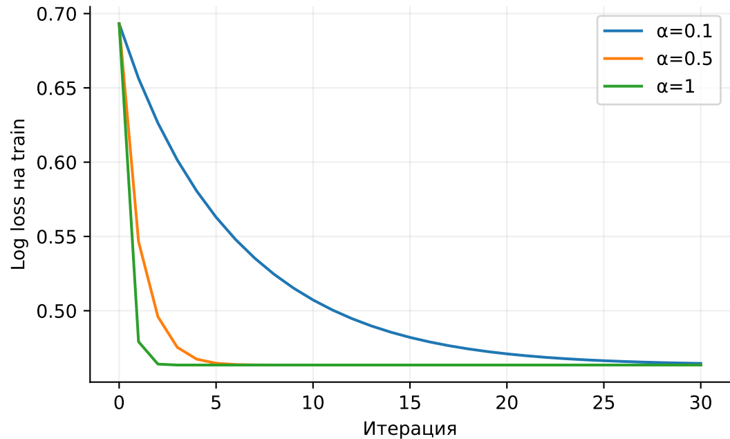
Метод Ньютона
